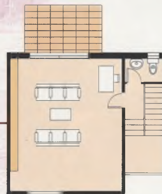
Planta Sota Coberta
