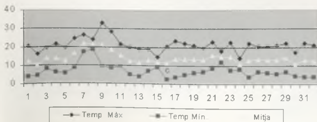
Evolució temperatures del 15 de març al 15 d'abril
