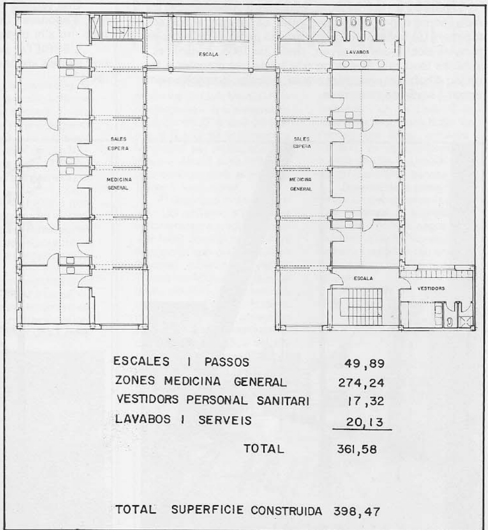
PLANTA SEGONA
