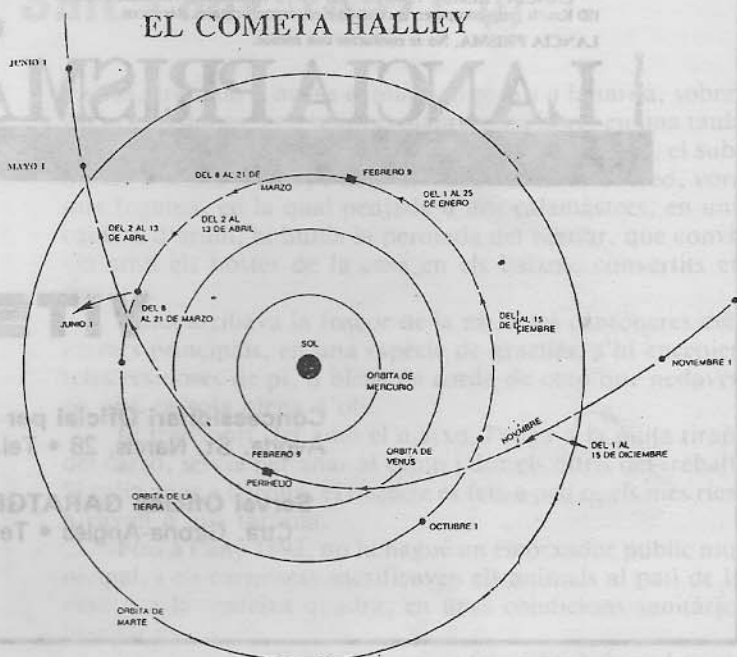
Situació del Cometa Halley, als voltants del centre del nostre sistema solar.
