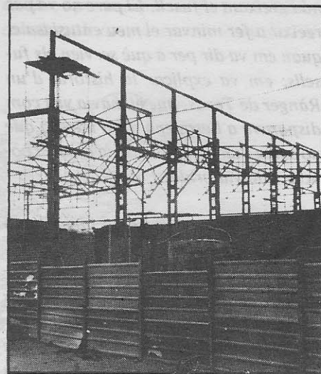
Començament del Pavelló... Vista estructura metàl·lica (Abril-85).
